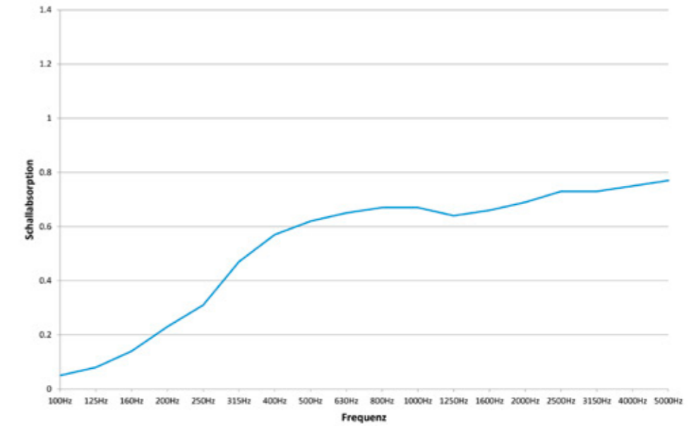
Schallabsorptionsgrad nach ISO 354 Messung der Schallabsorption in Hallräumen
